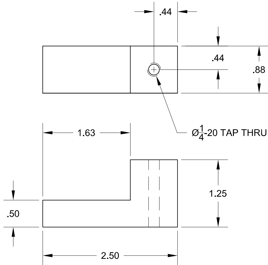
ITEM 2 SCALE 1:1
