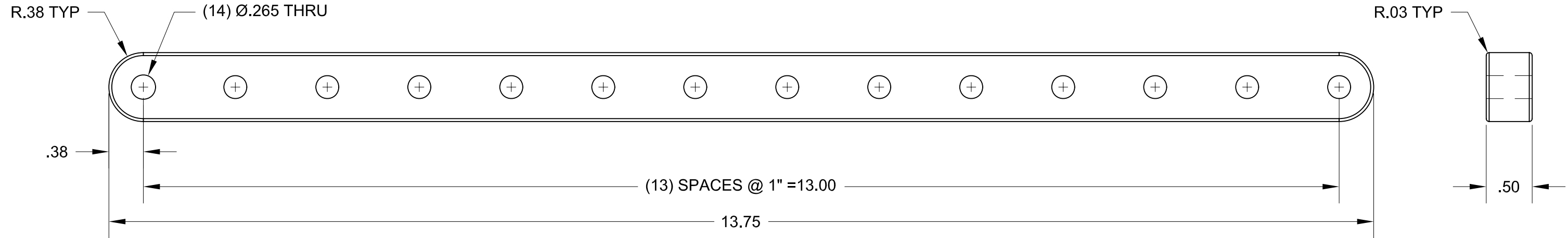
ITEM 1 SCALE 1:1
